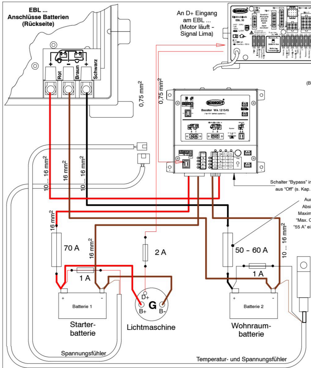
Bild 6 Fahrzeuge mit Schaudt EBL ... - Masseverbindung am Booster
